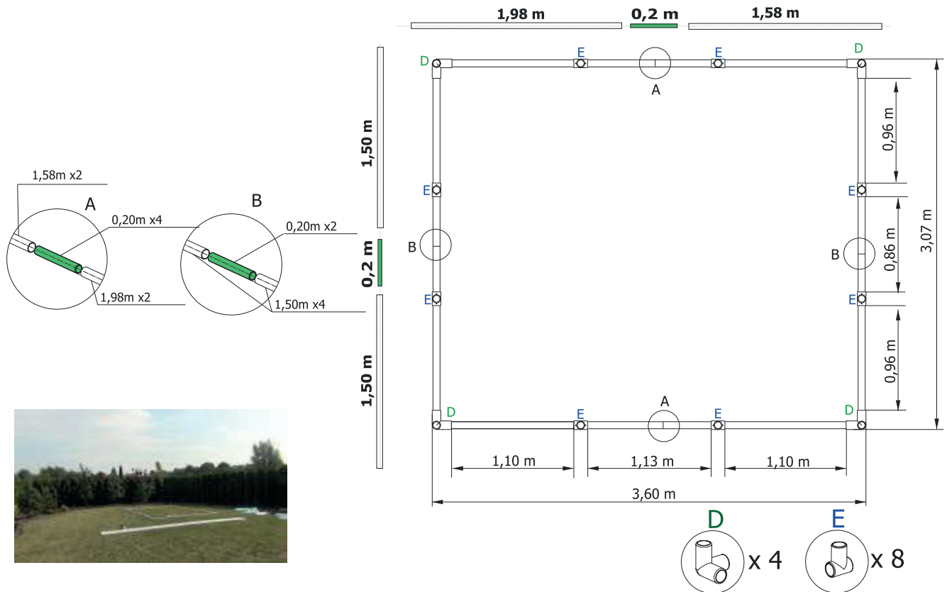
Scheme 2a
